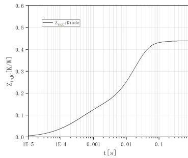
瞬态热阻抗 二极管, D5-D6 transient thermal impedance Diode, D5-D6
